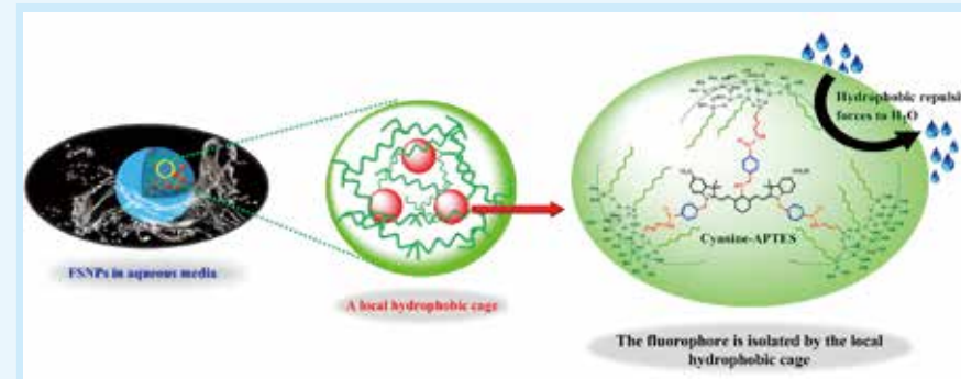
FSNPs 内部有机荧光染料的封装方式和“纳米疏水笼”结构
